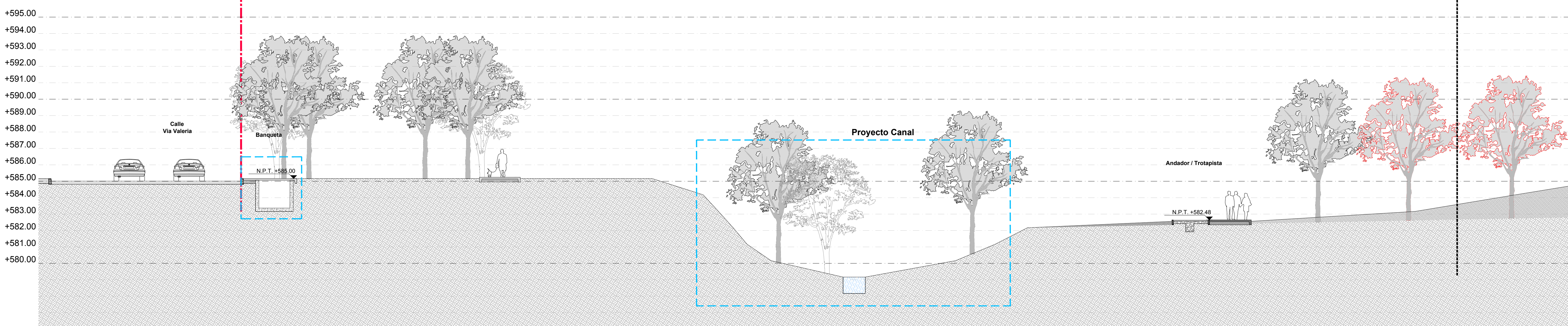
Tramo 01 - Corte 4
